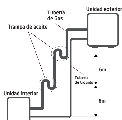
2. La unidad exterior está instalada más alta que la unidad interior
